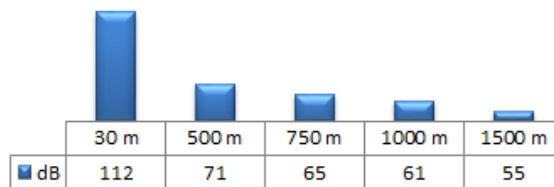
Zasięg akustyczny przy średnim poziomie hałasu (70 dB) panującym w mieście i dookólnym rozstawieniu głośników (180°)
