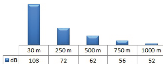
Zasięg akustyczny przy średnim poziomie hałasu (70 dB) panującym w mieście i dookólnym rozstawieniu głośników (180°)
